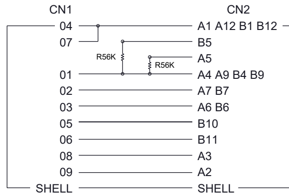
WIRING MAP
