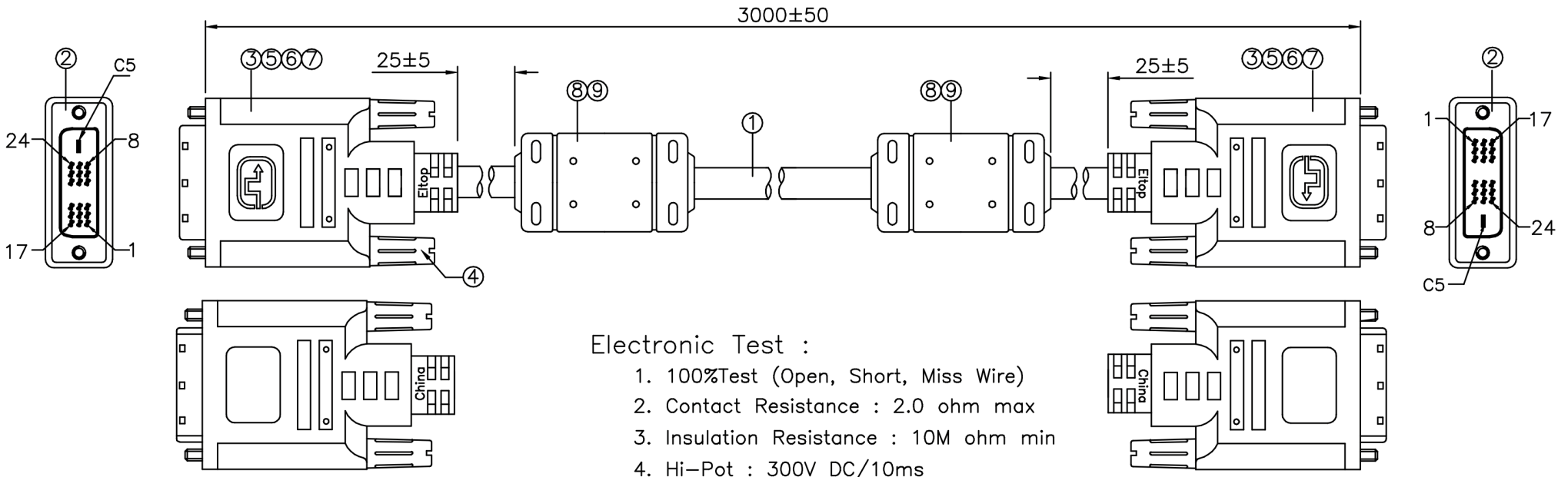
Conn.1 DVI-D Single Link Male
