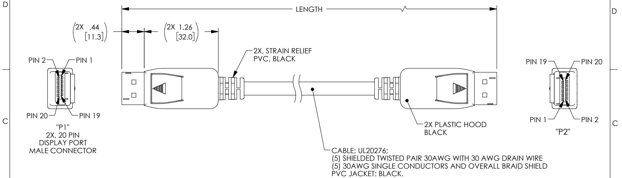
WIRING MAP B
