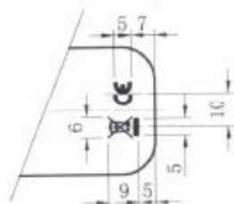
底面移印示意图
